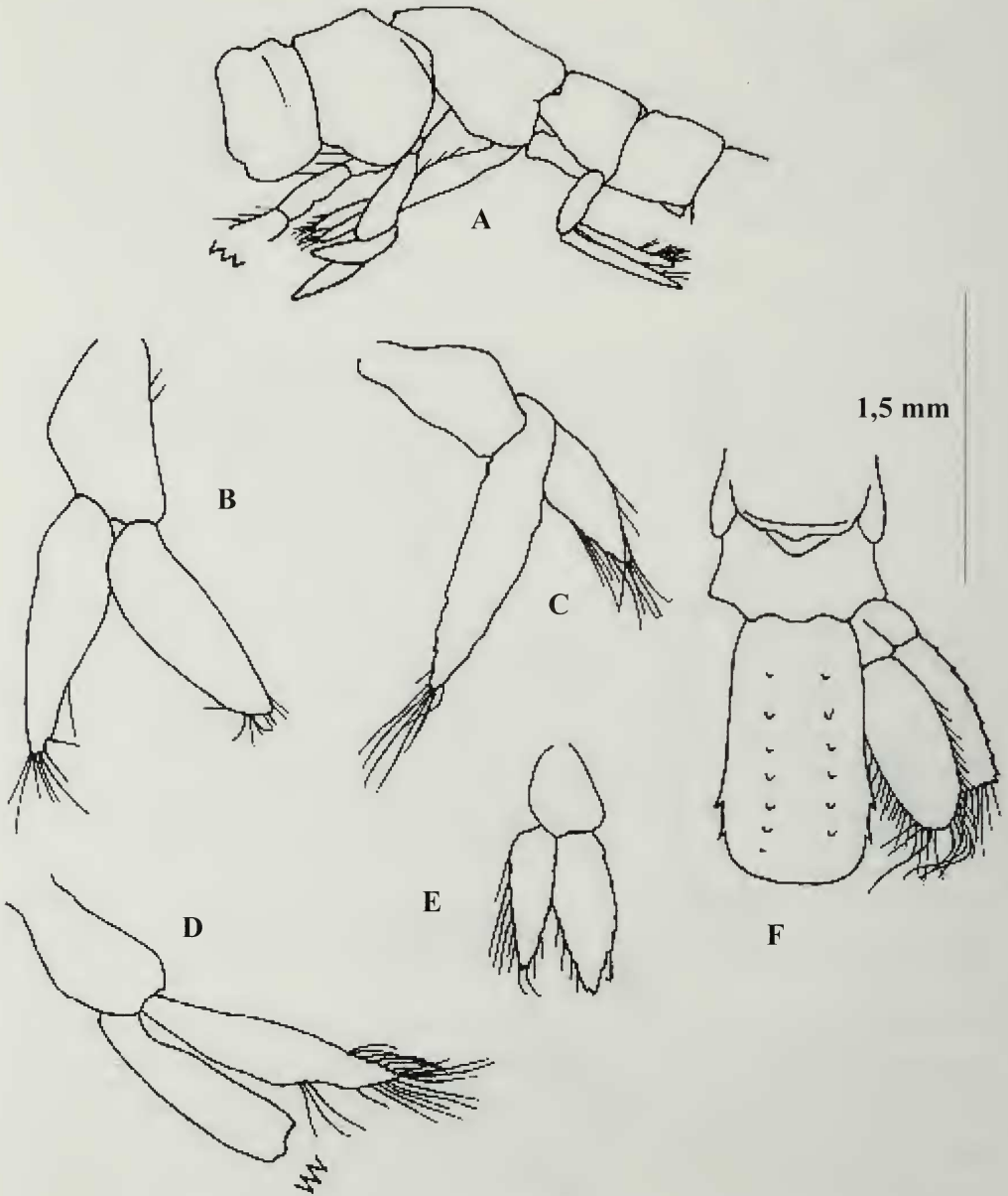
Figura 2. Spongiocaris goyi , especie nueva, A, vista lateral de los segmentos abdominales 1-5, B, pleópodo 2, C, pleópodo 3, D, pleópodo 4, E, pleópodo 5, F telson y urópodo derecho.
